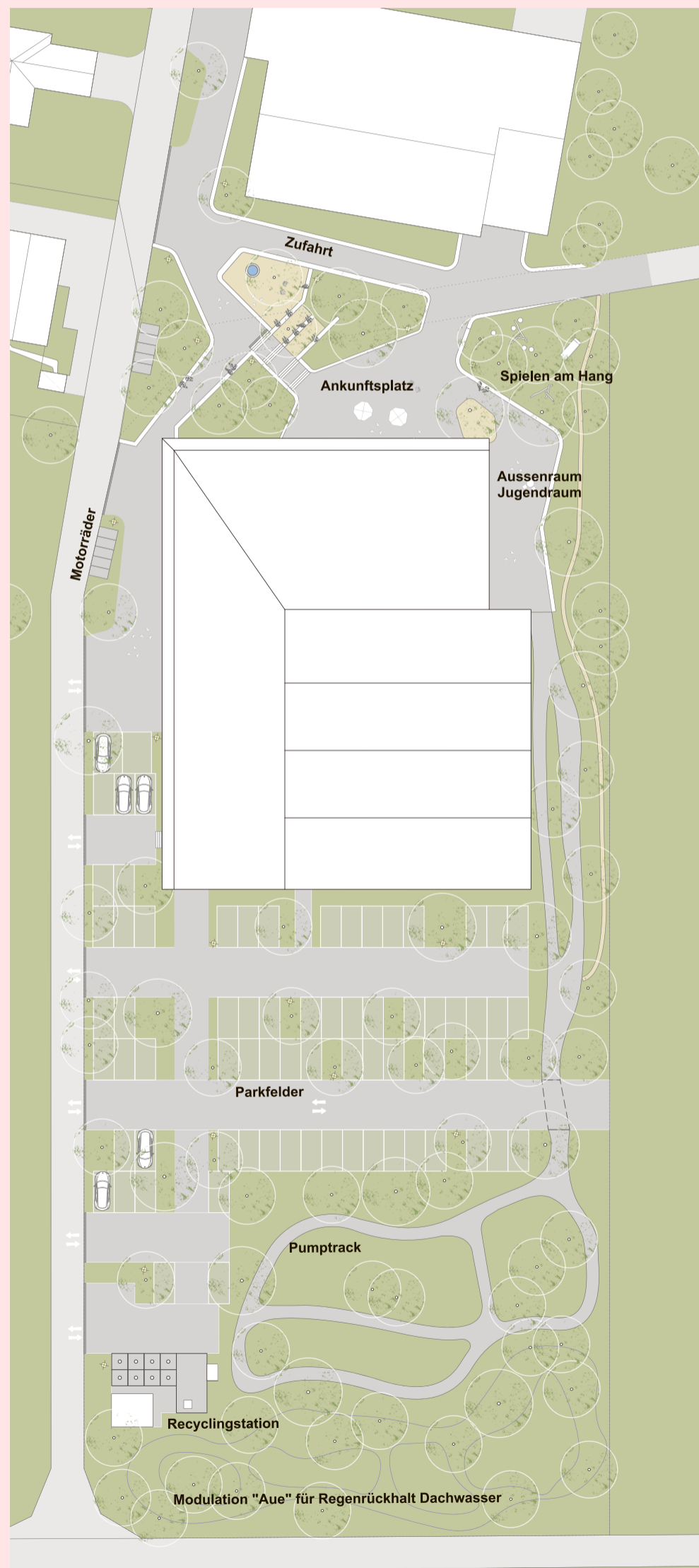
Mehrzweckhalle Breite, Situationsplan mit Dachaufsicht
